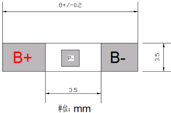
301030 保护板装配图
