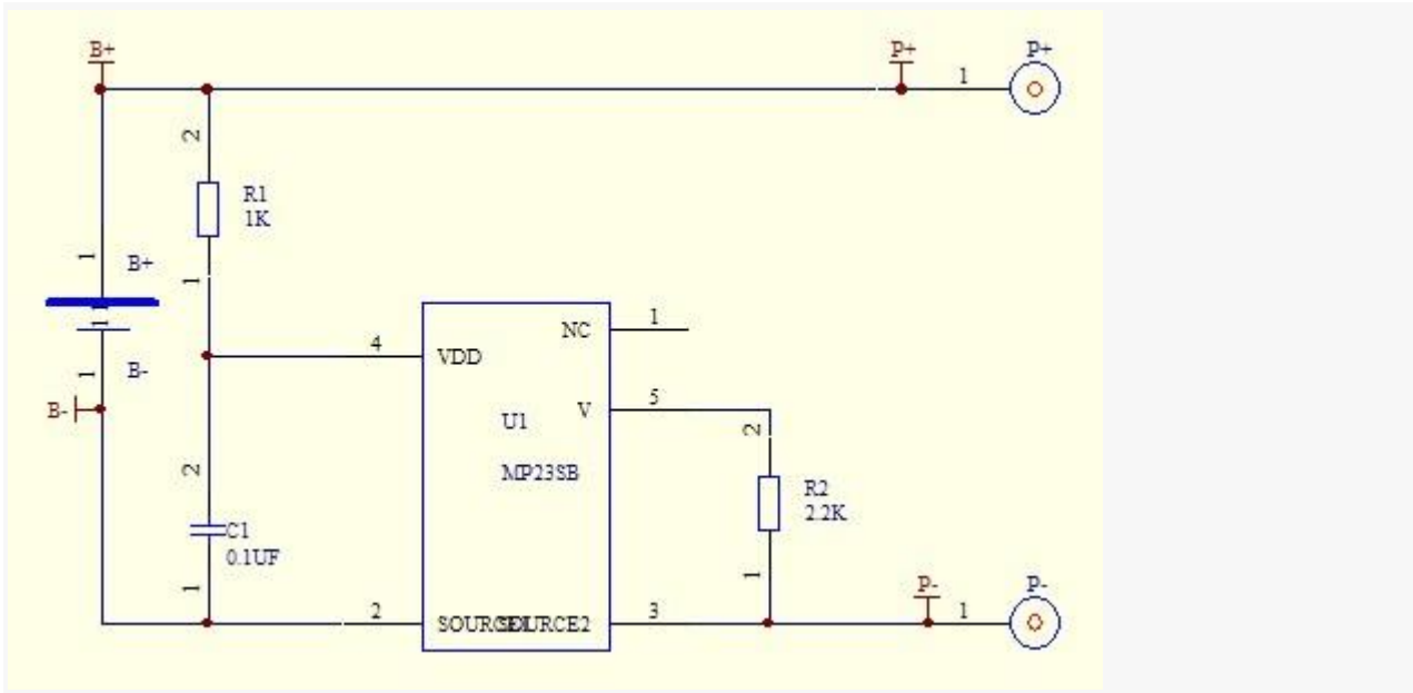
线路板原理图
